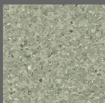
004 - Asparagus - LRV-37
