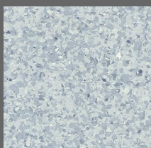
005 - Ladoga - LRV-46
